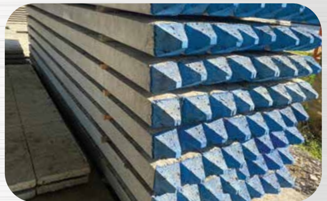
เสาเข็มคอนกรีตอัดแรง Concrete piles
